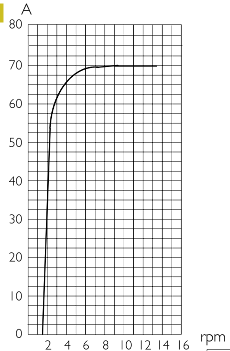
CURVA DI EROGAZIONE CORRENTE ALTERNATORE
